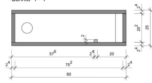
Schnitt 1 - 1
