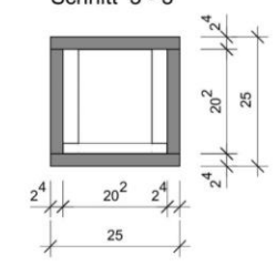
Schnitt 3 - 3
